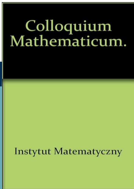
Colloquium Mathematicum
