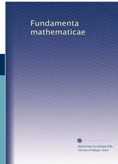
Fundamenta Mathematicae
