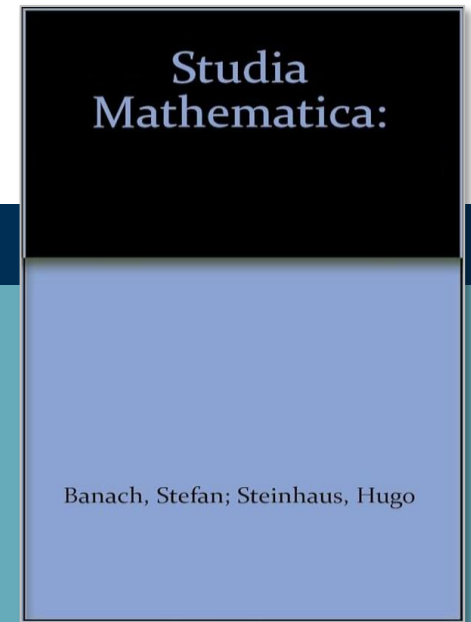
Studia Mathematica
